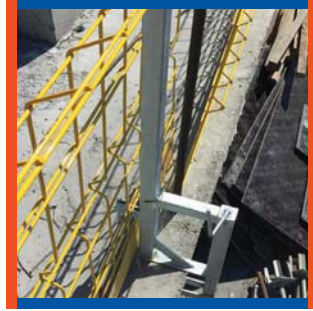
Kiriş Sıkıştırılmalı Dikme Beam Compressible Post Poste à Poutre Compressible
